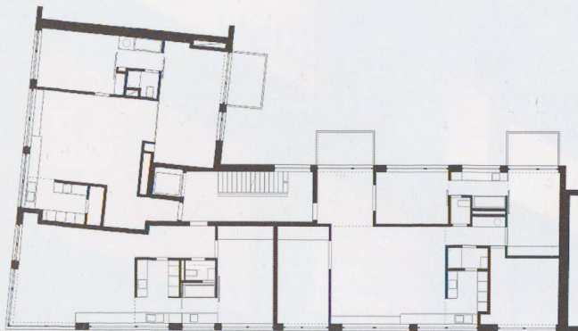
Pianta primo e secondo piano
